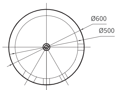
Pohled shora
