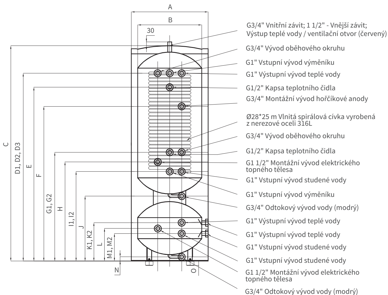
4 - Ø60 plastové nohy (podpěry)
