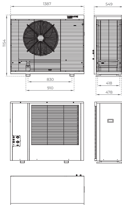
Gesamtabmessungen der Wärmepumpe TH-R290-S10-3P | 10 kW
