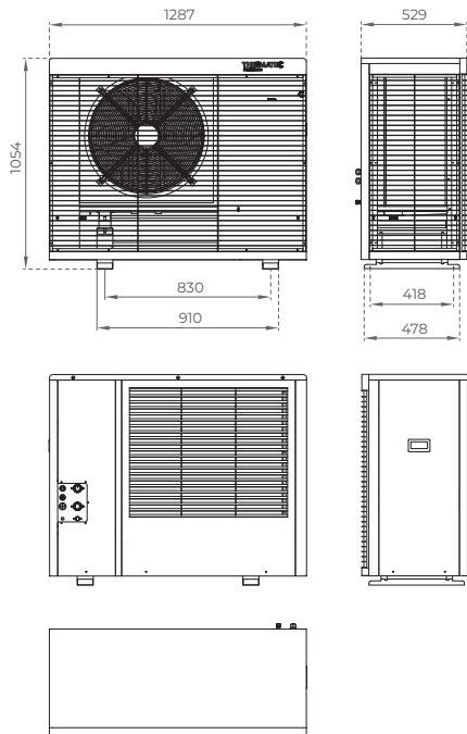
Gesamtabmessungen der Wärmepumpe TH-R290-S06-1P | 6 kW
