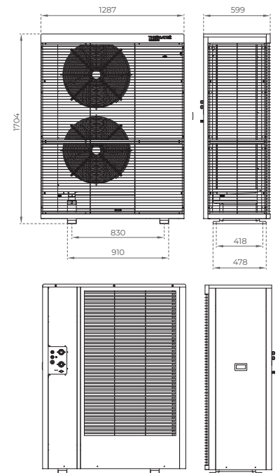
Gesamtabmessungen der Wärmepumpe TH-R290-S16-3P | 16 kW
