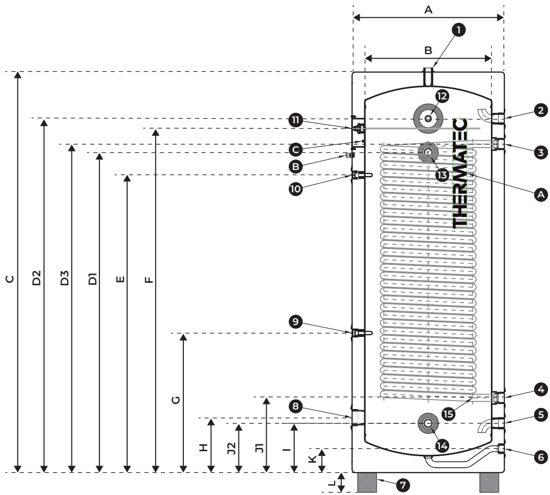
Rysunek zbiornika zbiornika C.W.U. 200L ULTIMATE AQUA z pojedynczą wężownicą
