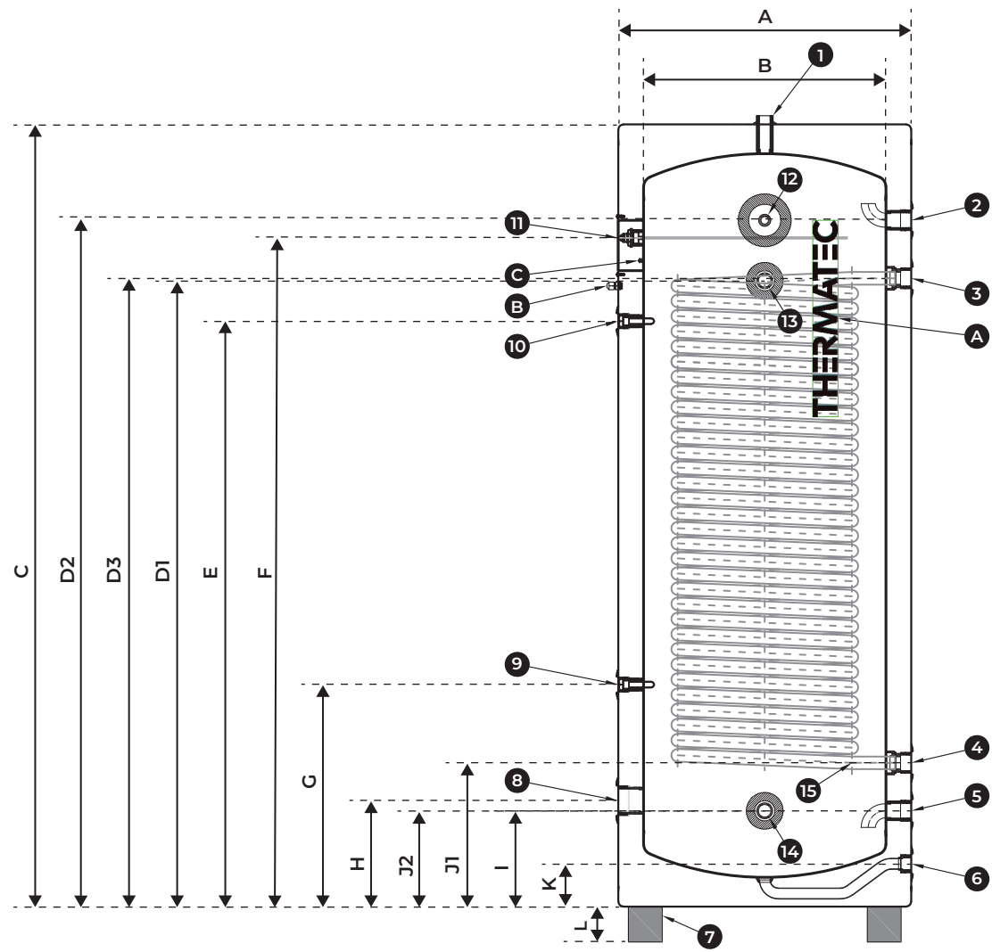
Rysunek zbiornika zbiornika C.W.U. 250L ULTIMATE AQUA z pojedynczą wężownicą
