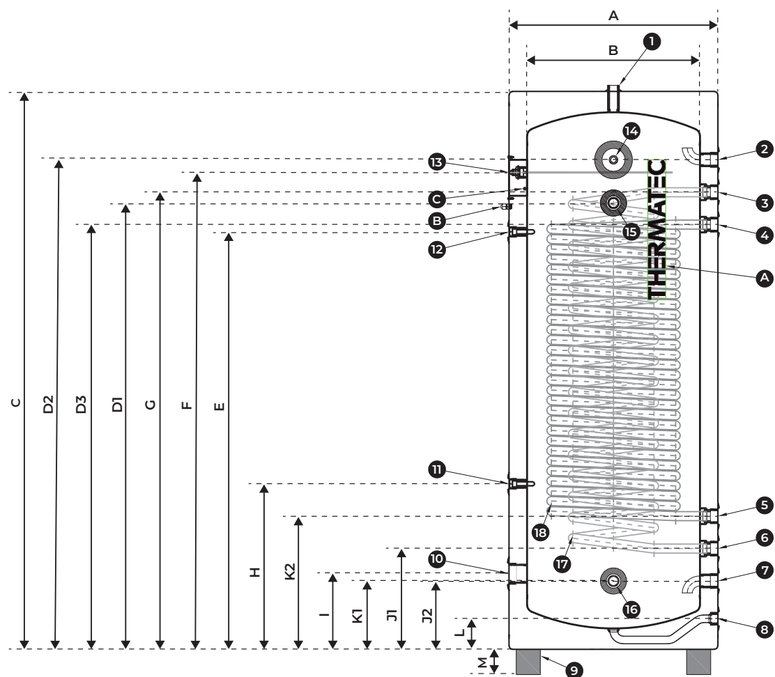
Rysunek zbiornika zbiornika C.W.U. 250L ULTIMATE AQUA z podwójną wężownicą
