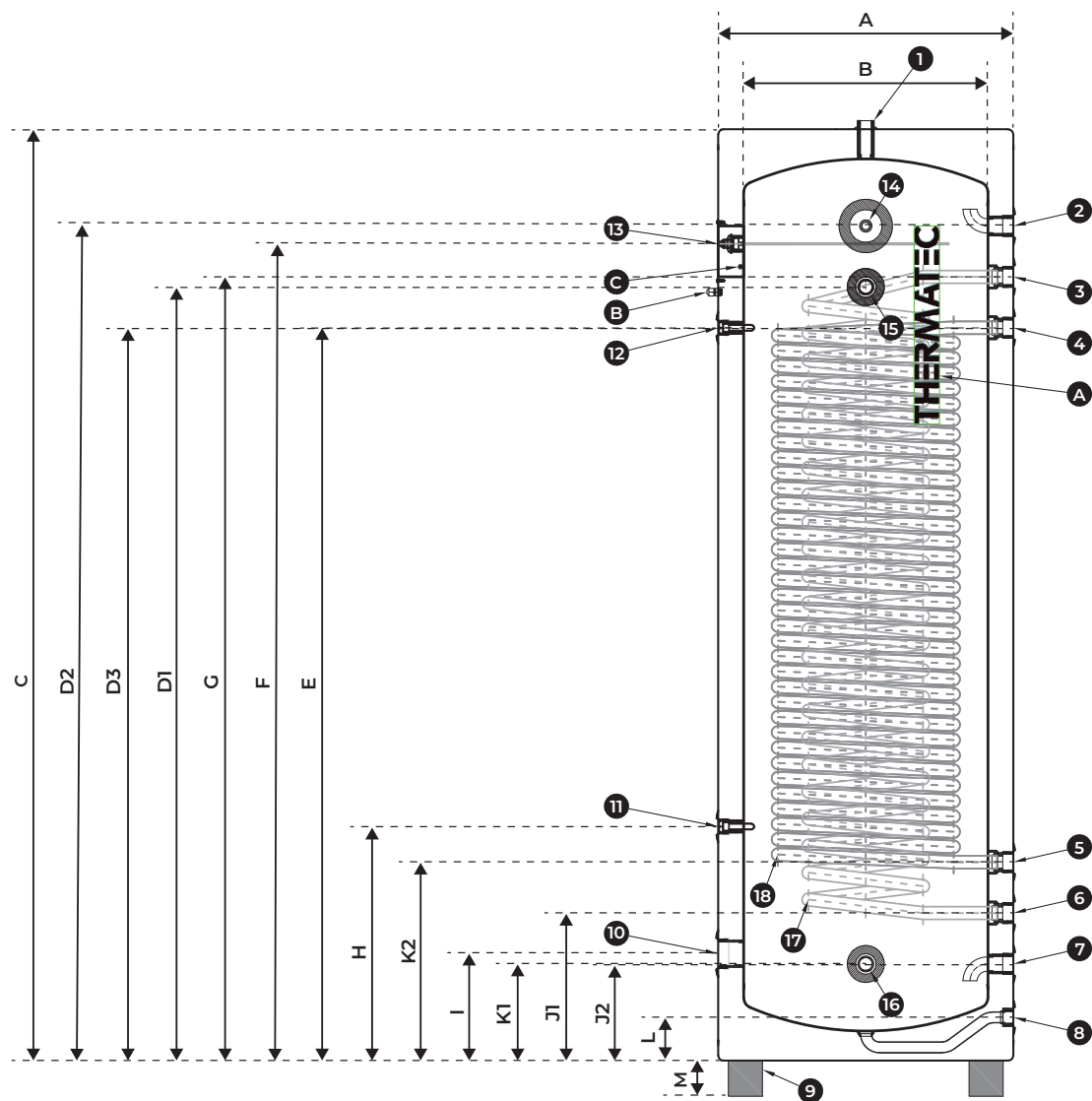
Rysunek zbiornika zbiornika C.W.U. 300L ULTIMATE AQUA z podwójną wężownicą
