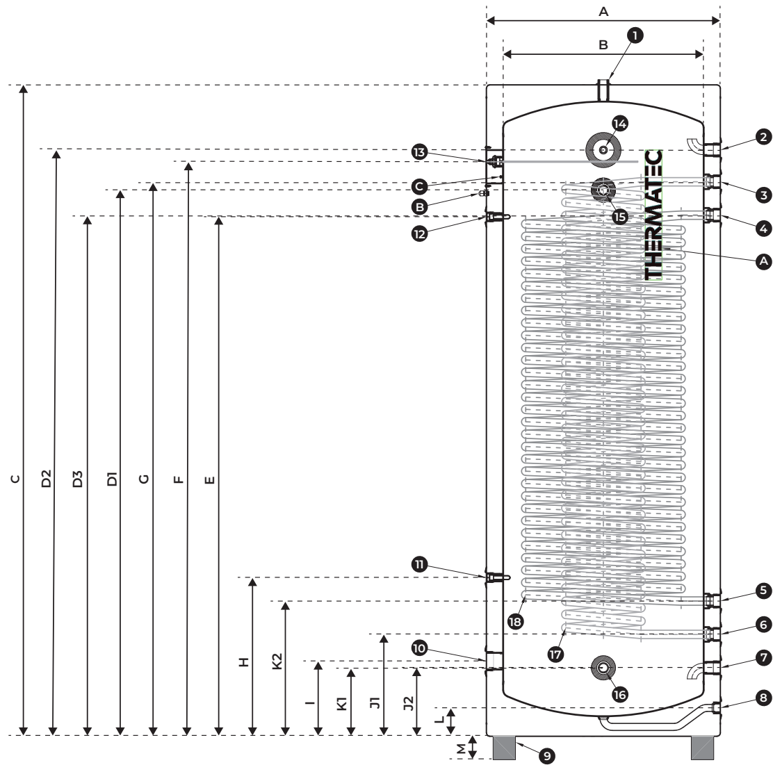
Rysunek zbiornika C.W.U. 500L ULTIMATE AQUA z podwójną wężownicą
